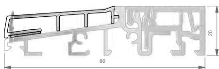
Nakładka odwadniająca z aluminium (TSA...), 1950 mm, wyrównująca poziom posadzki, samoprzylepna
