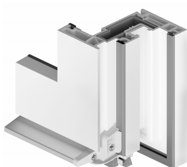
okapnik z zakończeniem okapnika skrzydła czynnego
