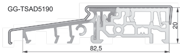
Nakładka ochronna prog, PCV szary, L = 980 mm
