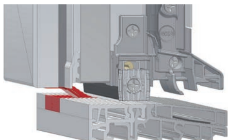
Stoper skrzydła biernego SAFE STP
