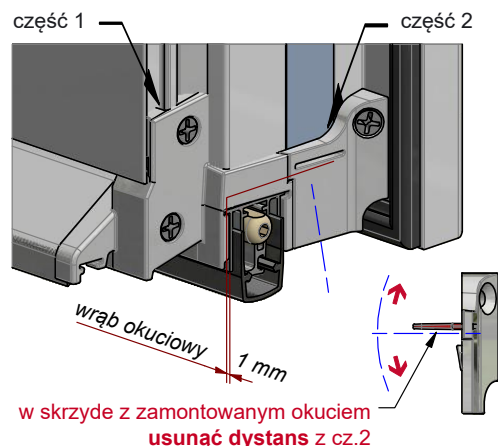
GG-EK-BDA8531- strona zamykająca
