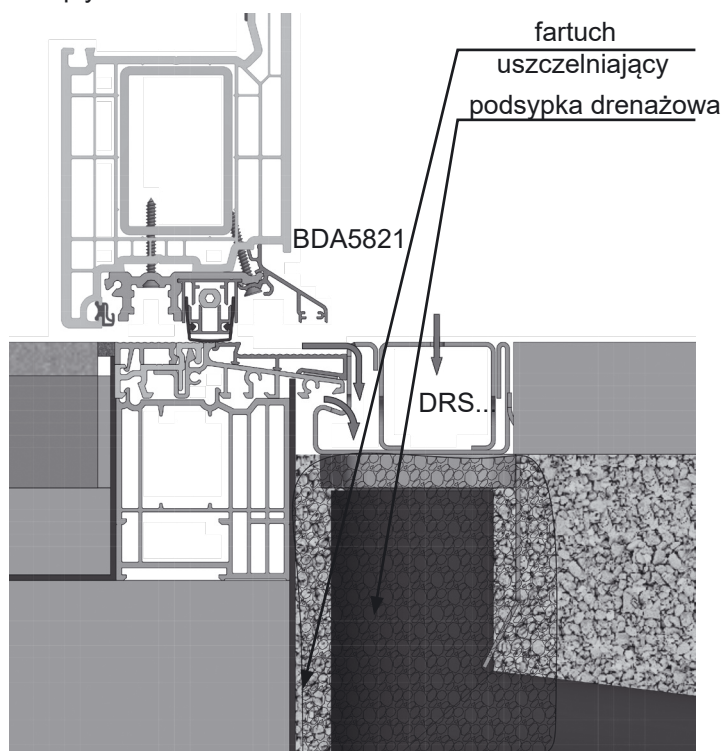
DRS1250/DRS1970 z odpływem Ø50
