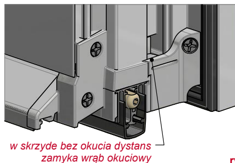
GG-EK-BDA8531- strona zawiasowa
