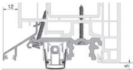
Profil ALU okapnika PLAN, L=1970 mm
