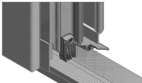
Łącznik ruchomego słupka, wkręty INOX 3,5 x 19 mm
